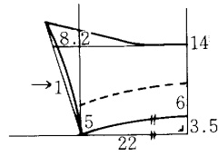
製図 コート
